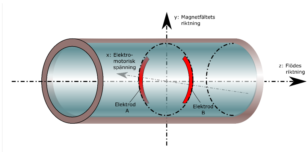
Figur 15. Induktiv flödesmätare
