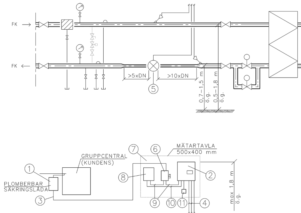
Figur 19. Komponenter i kylcentral
