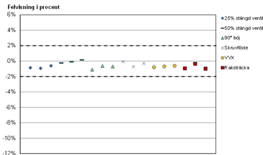
Figur 14. Flödesgivare godkänd vid alla placeringar direkt efter störningar eller ostörd raksträcka
