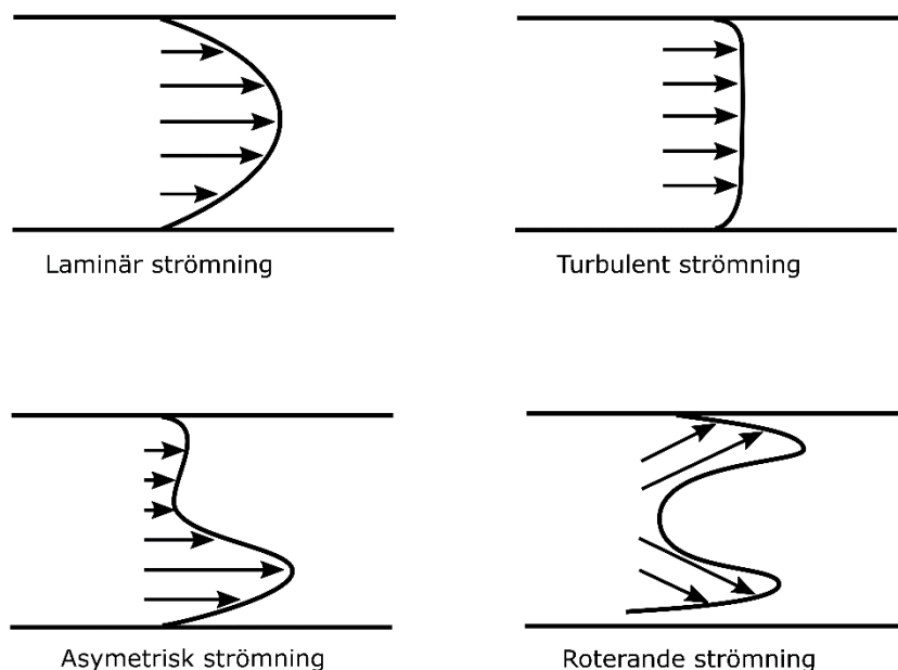
Figur 11. Olika flödesprofiler
